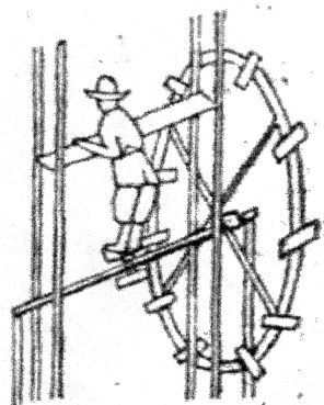
Рис. 2. «Аяк-Чигирь — ножной чигирь, применяемый в Кайдаульской волости Тургайского уезда (в верховьях Джиланчика)» [28]
